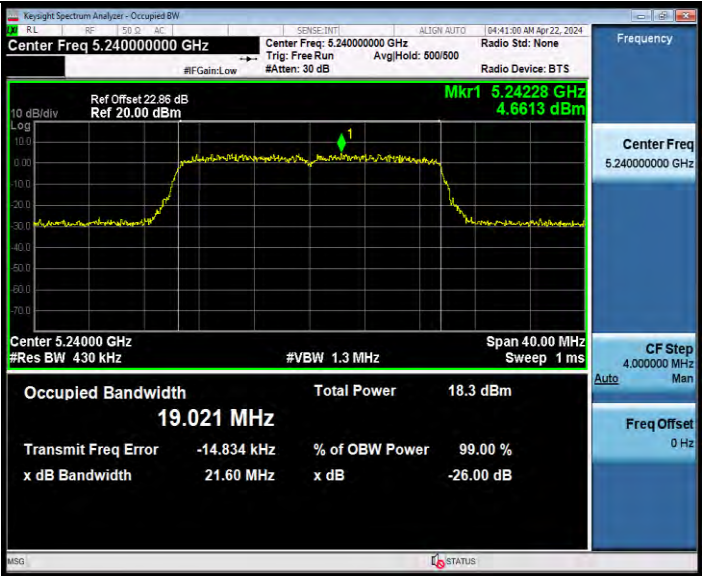
11AX20MIMO_Ant9_5240
