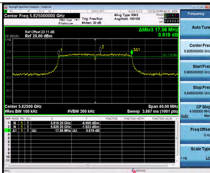
11N20MIMO Ant9 5825
