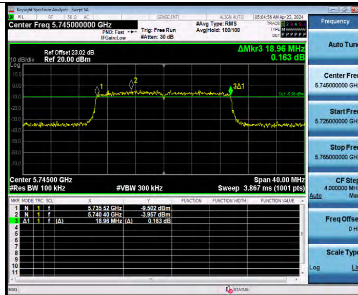
11AX20MIMO_Ant9_5745
