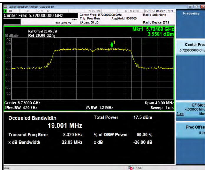
11AX20MIMO_Ant9_5720
