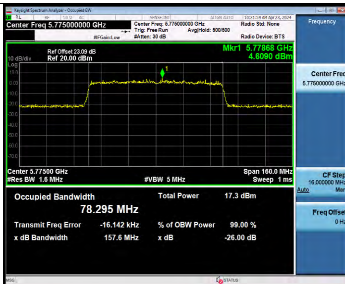
11AX80MIMO_Ant9_5775
