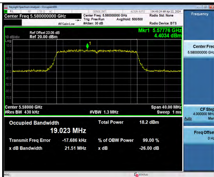
11AX20MIMO_Ant9_5580
