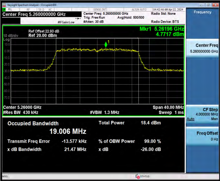
11AX20MIMO_Ant9_5260
