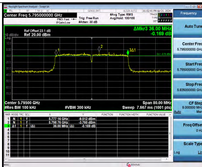
11N40MIMO_Ant9_5795
