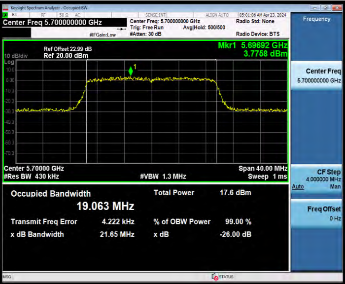
11AX20MIMO_Ant9_5700
