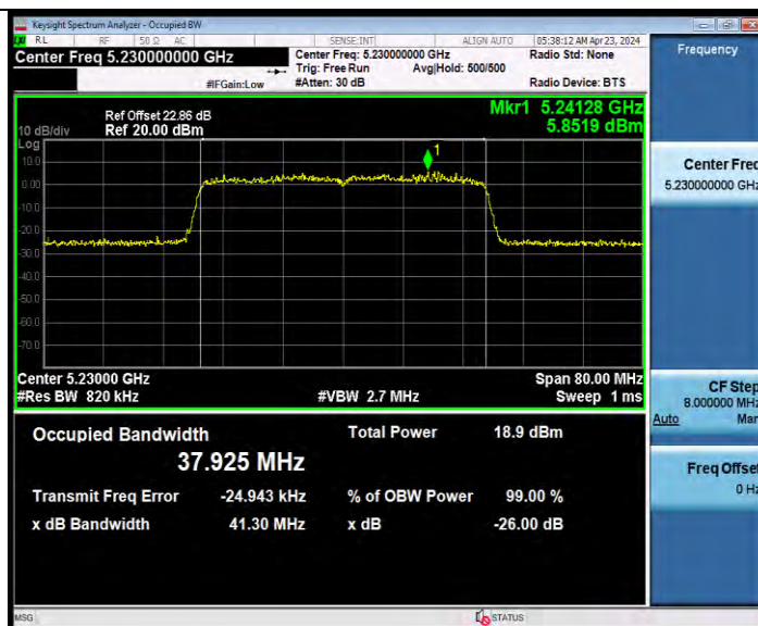
11AX40MIMO_Ant9_5230
