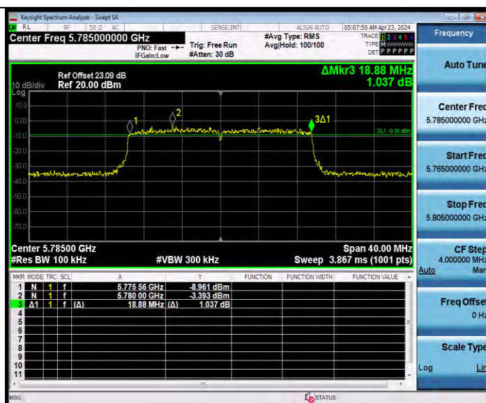
11AX20MIMO_Ant9_5785
