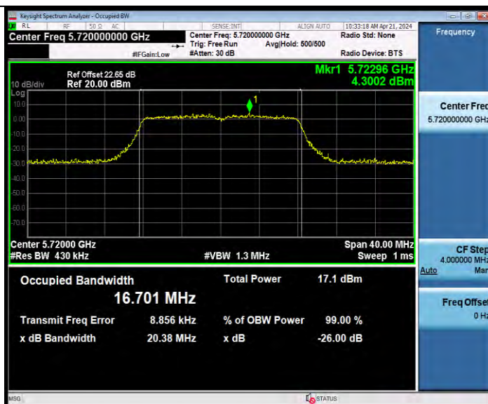
11A-CDD Ant9 5720
