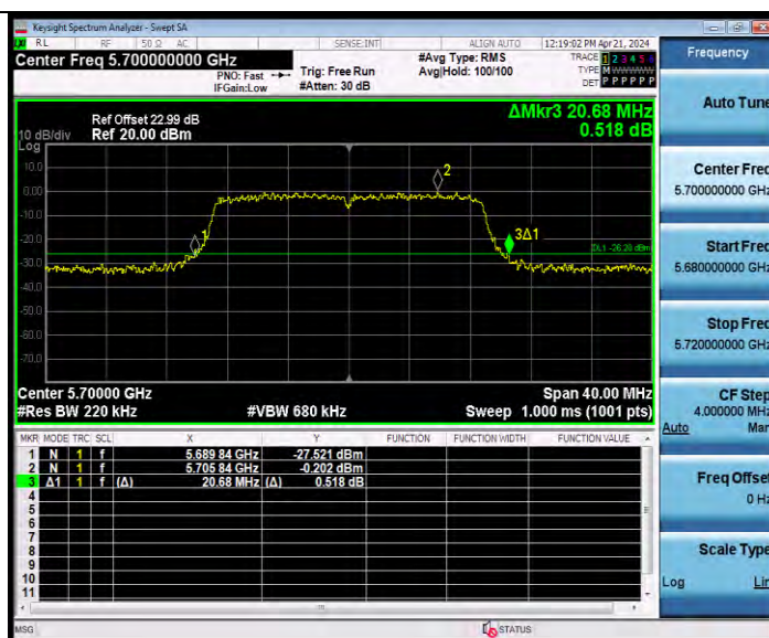
11N20MIMO Ant9 5700
