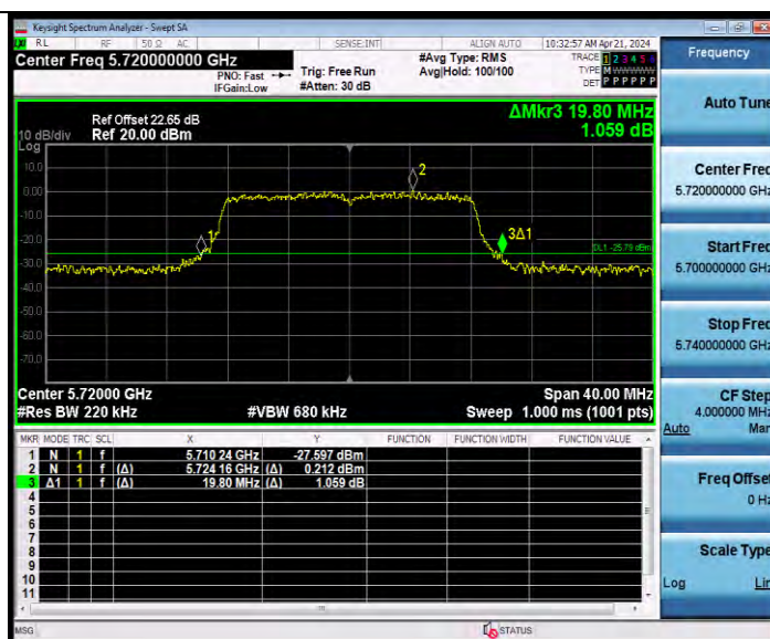
11A-CDD Ant9 5720
