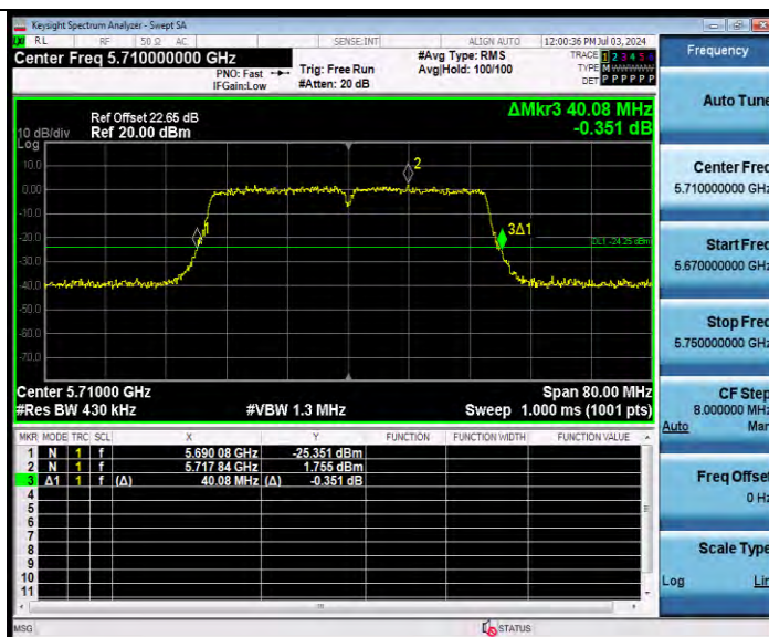
11N40MIMO Ant9 5710
