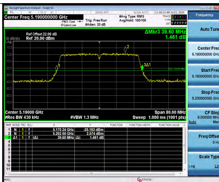
11N40MIMO Ant9 5190
