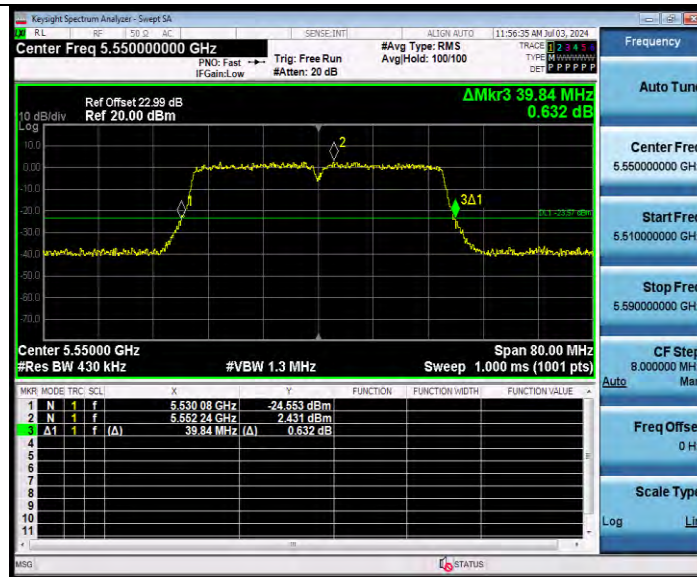
11N40MIMO Ant9 5550
