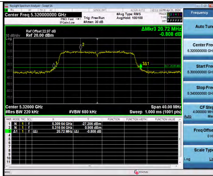
11N20MIMO Ant9 5320
