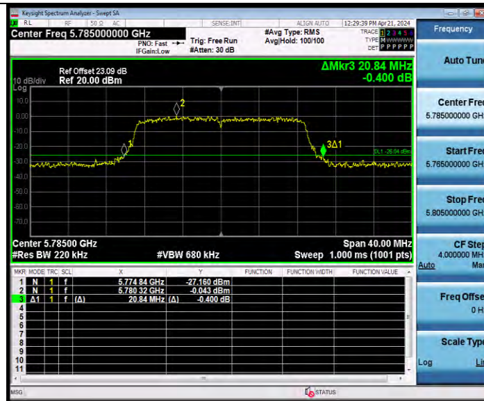
11N20MIMO Ant9 5785
