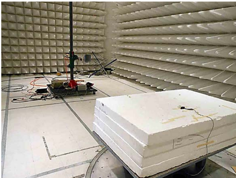
12-18GHz
