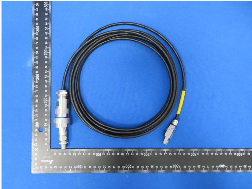
(13) EUT Photo - EUT Power Cable
