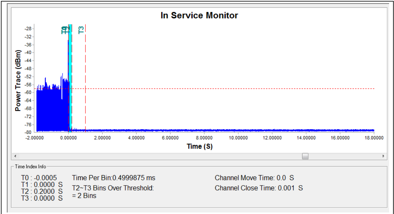
(5270MHz, 802.11n (HT40))
