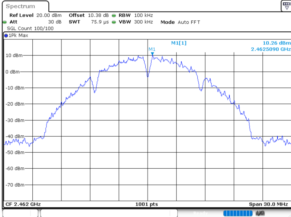
Band Edge NVNT b 2462MHz Ant 4 Emission
