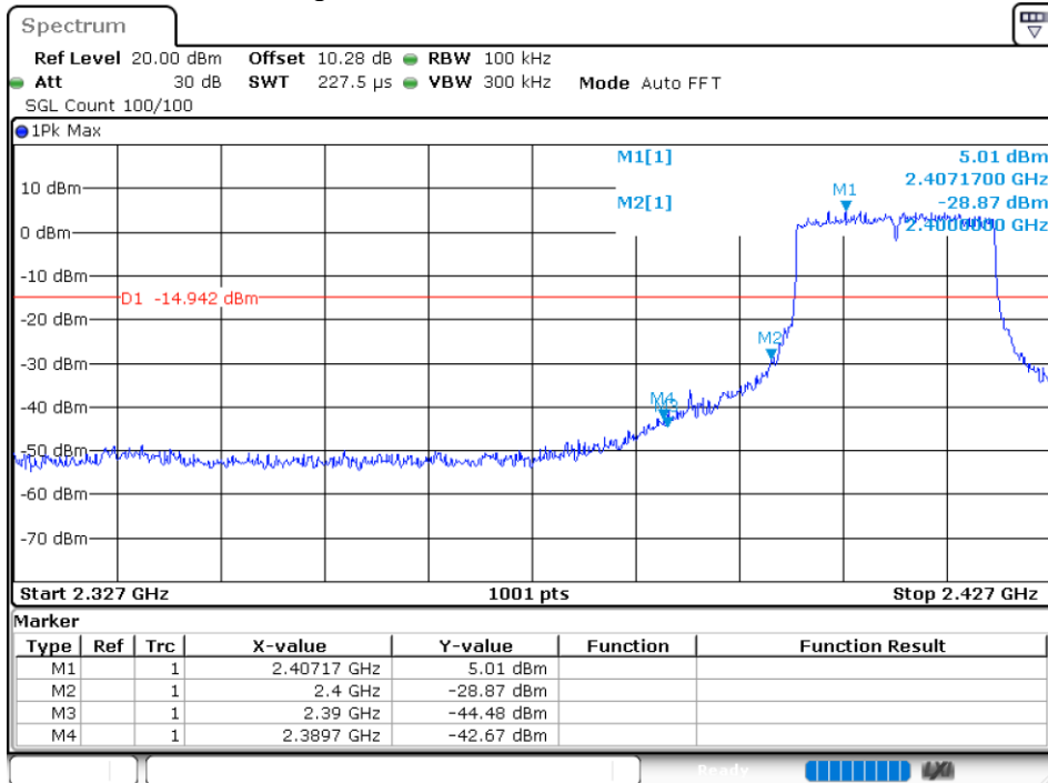
Band Edge NVNT ax20 2412MHz Ant 4 Emission
