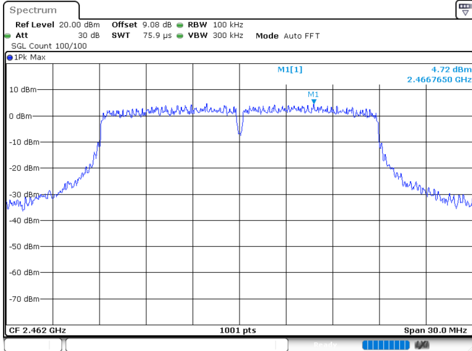
Band Edge NVNT n20 2462MHz Ant 3 Emission
