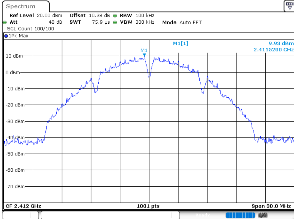
Band Edge NVNT b 2412MHz Ant 4 Emission
