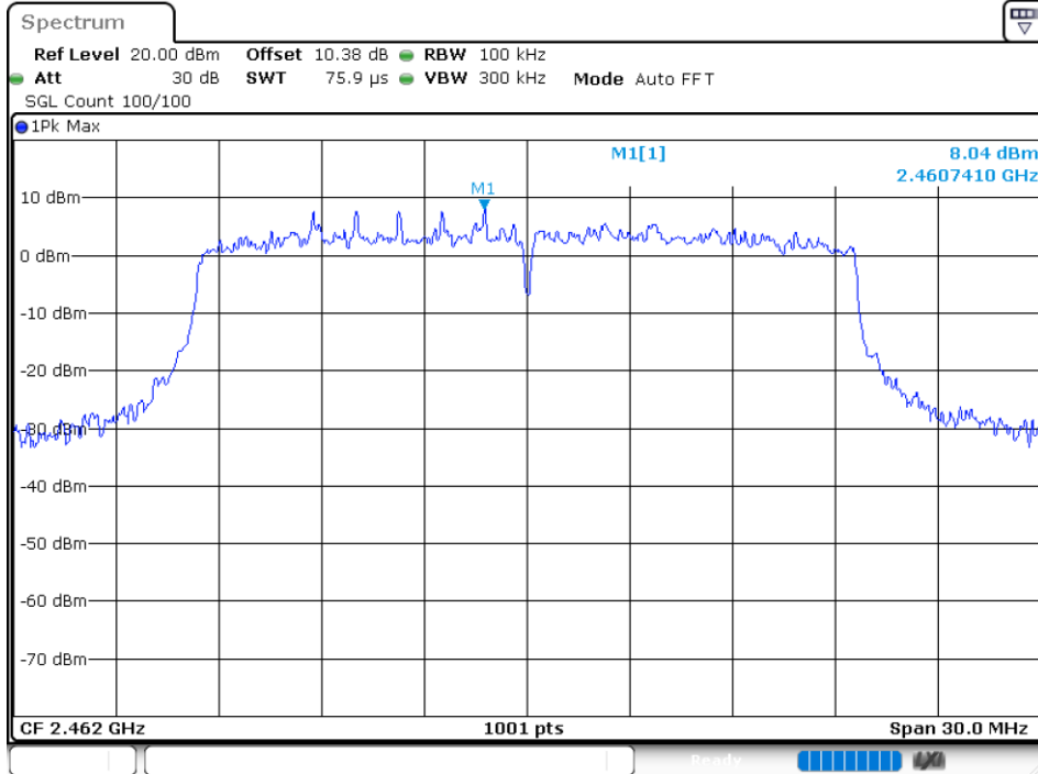
Band Edge NVNT ax20 2462MHz Ant 4 Emission
