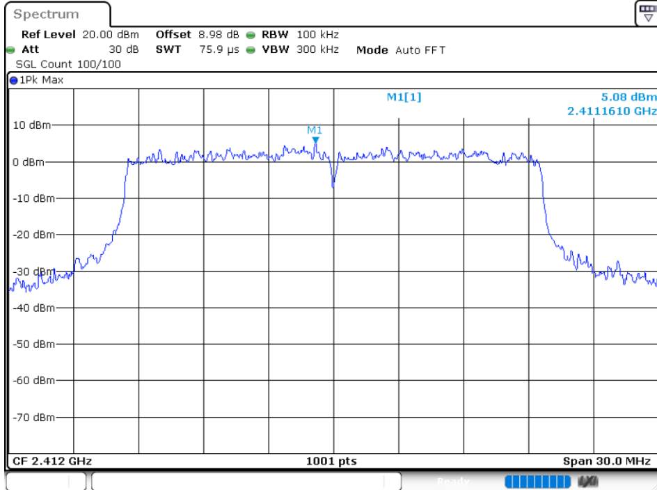
Band Edge NVNT ax20 2412MHz Ant 3 Emission
