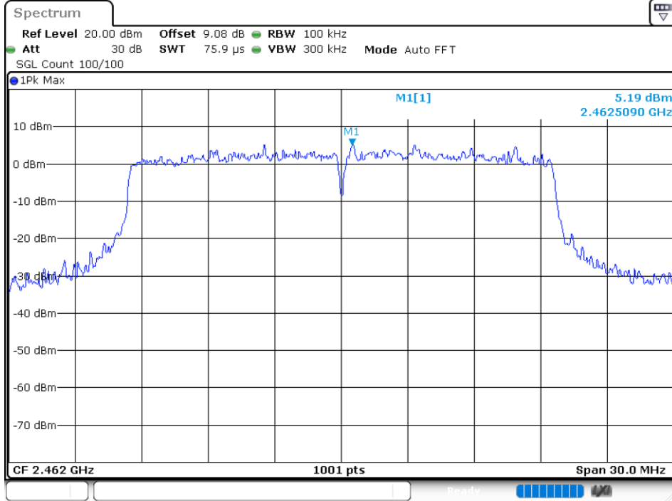
Band Edge NVNT ax20 2462MHz Ant 3 Emission
