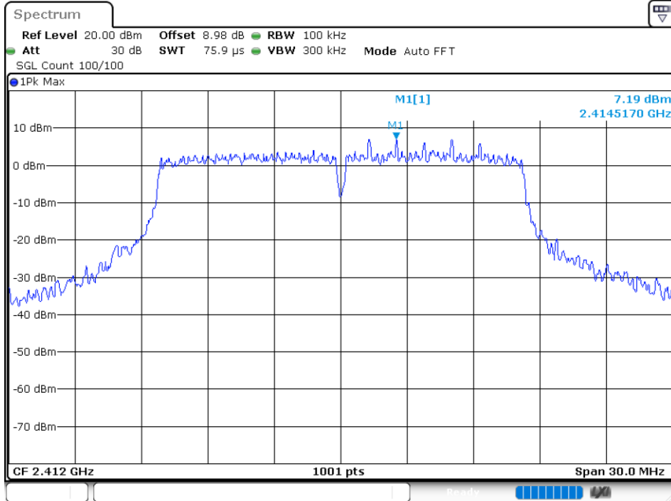
Band Edge NVNT g 2412MHz Ant 3 Emission
