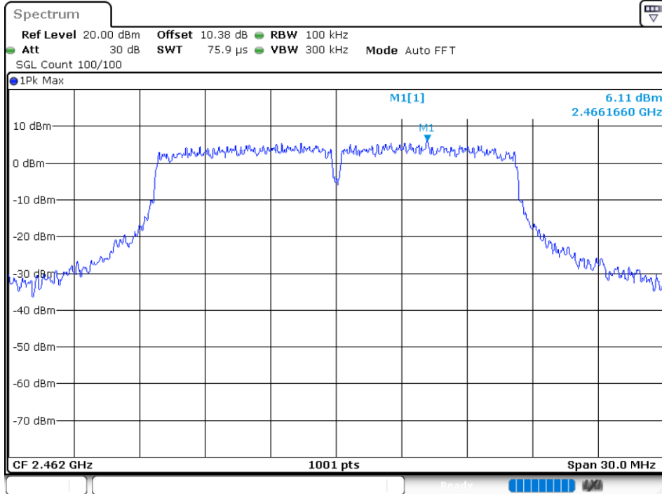
Band Edge NVNT g 2462MHz Ant 4 Emission
