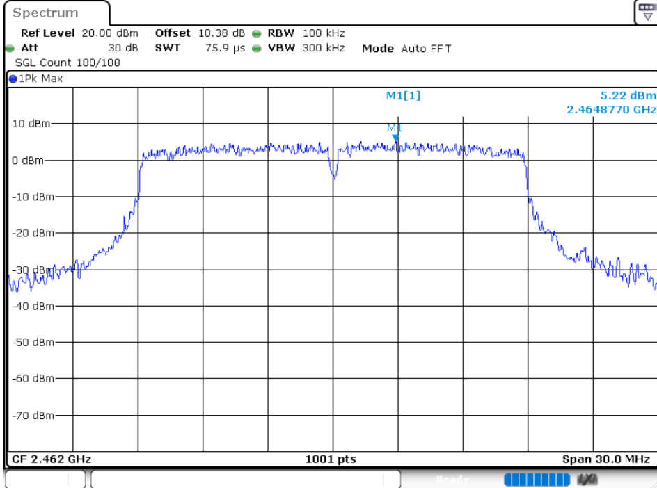
Band Edge NVNT n20 2462MHz Ant 4 Emission
