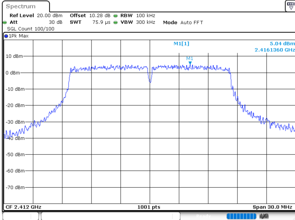
Band Edge NVNT g 2412MHz Ant 4 Emission
