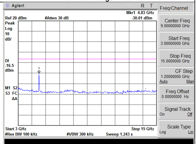
3GHz~15GHz
