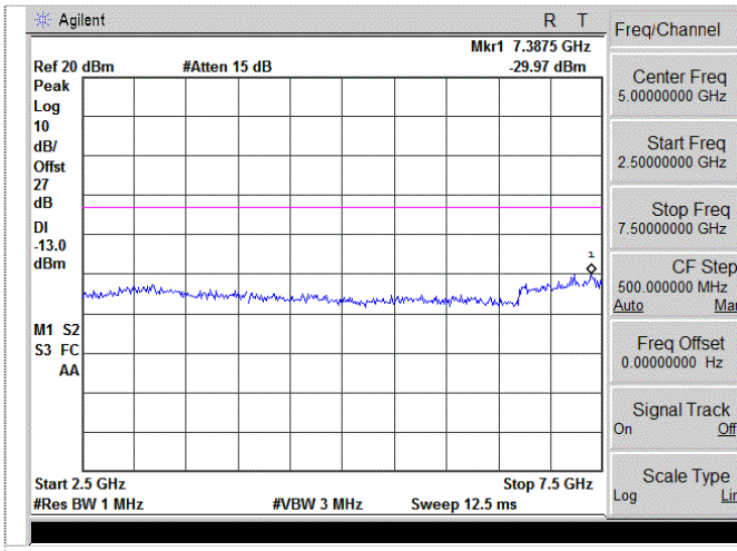
2.5GHz~7.5GHz
