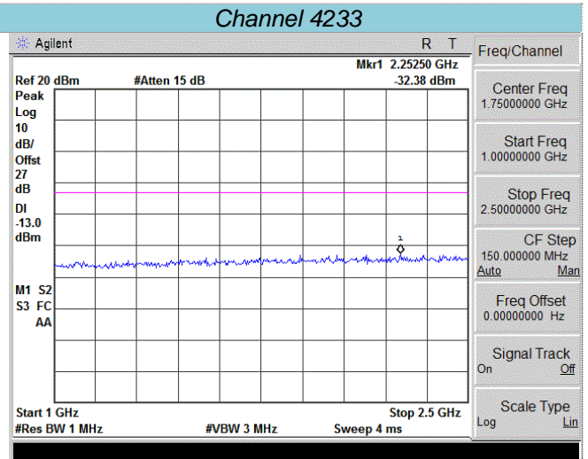
1GHz~2.5GHz
