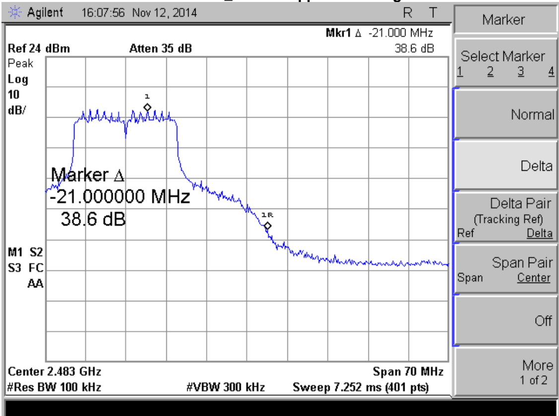
For 802.11n_20MHz: Upper Band Edge
