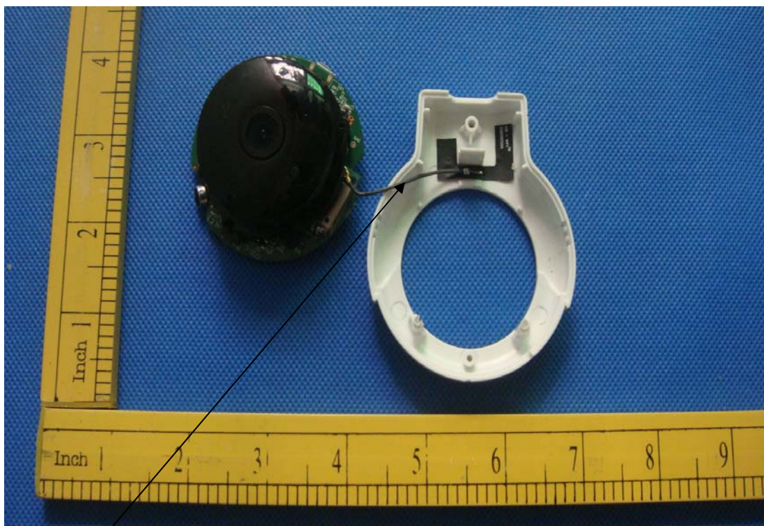
Antenna
