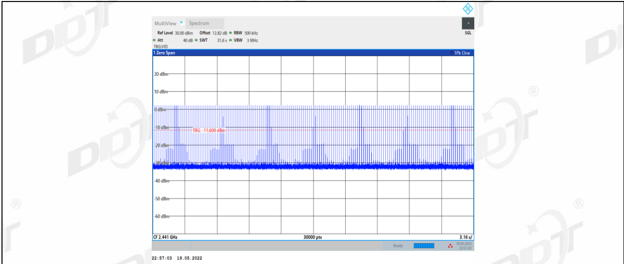
DH5_Ant1_Hop
