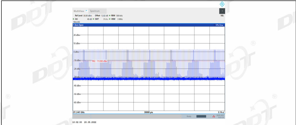
2DH5_Ant1_Hop
