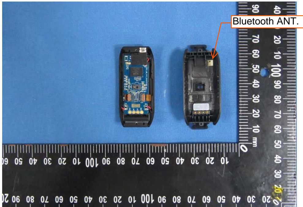
EUT Photo 2 )
