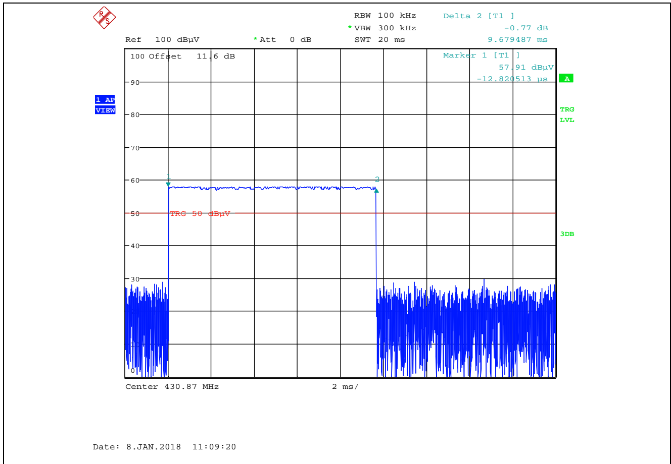
Plot 5.3.3.1.3. Duty Cycle (Pulse 1)
