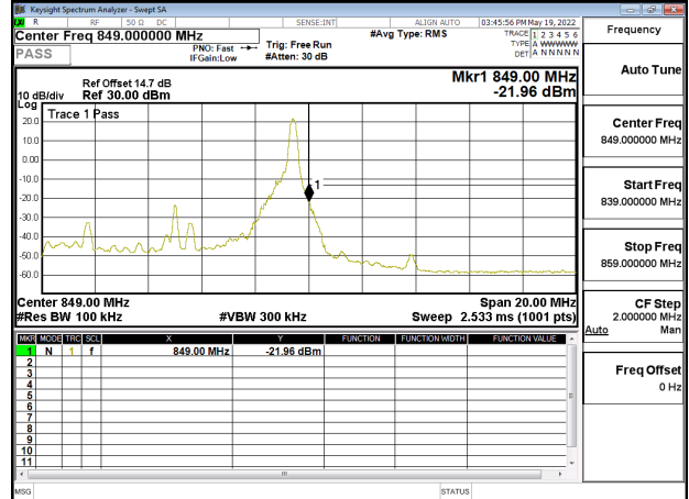
Band Edge_Band26_10MHz_QPSK_RB1_49_CH26990
