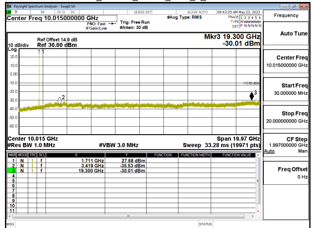
Band4_10MHz_QPSK_RB1_0_CH20175
