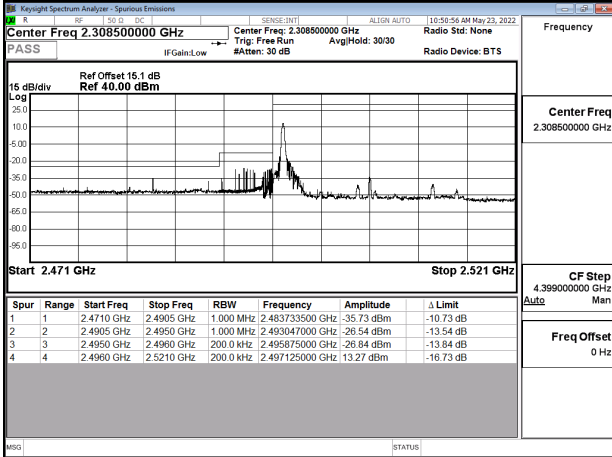
Emission Mask_Band41_20MHz_QPSK_RB1_99_CH41490
