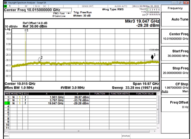
Band2_10MHz_QPSK_RB1_0_CH19150
