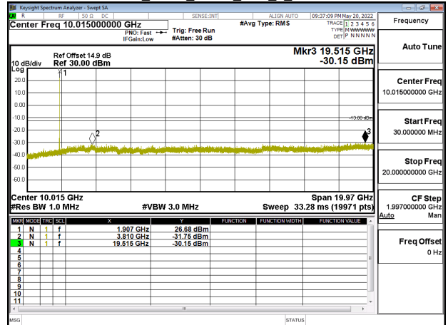
Band2_3MHz_QPSK_RB1_0_CH19185
