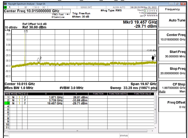
Band2_20MHz_QPSK_RB1_0_CH19100
