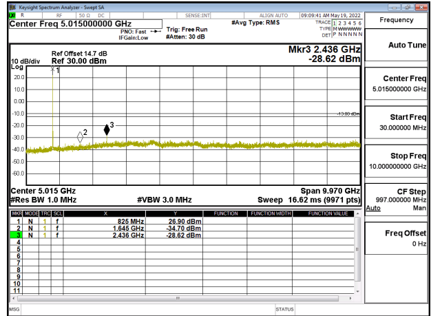
Band5_10MHz_QPSK_RB1_0_CH20525
