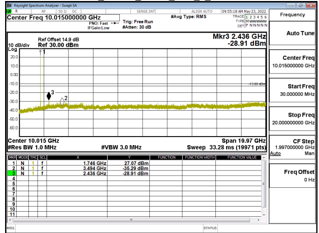
Band4_10MHz_QPSK_RB1_0_CH20350
