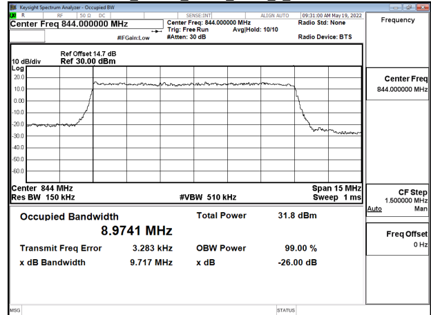
Band5_10MHz_QPSK_RB50_0_CH20600
