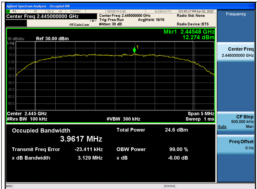
Test_Graph_GFSK_ANT1_2445_DTSBW
