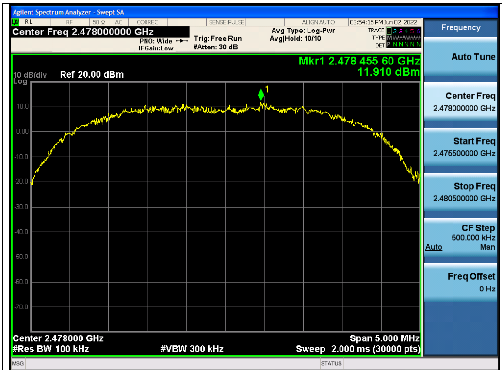
Test_Graph_GFSK_ANT1_2478_Reference Level
