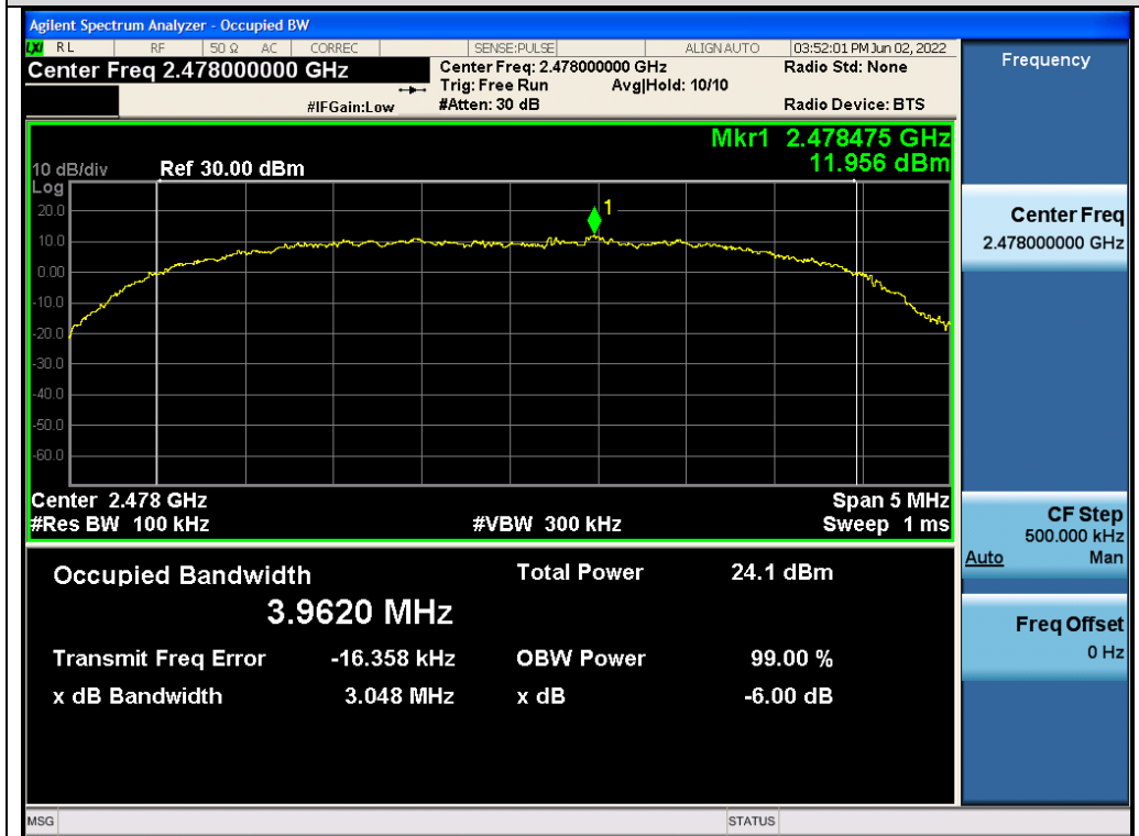
Test_Graph_GFSK_ANT1_2478_DTSBW
