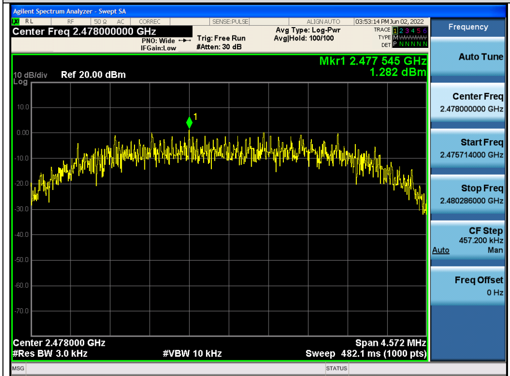
Test_Graph_GFSK_ANT1_2478_PSD
