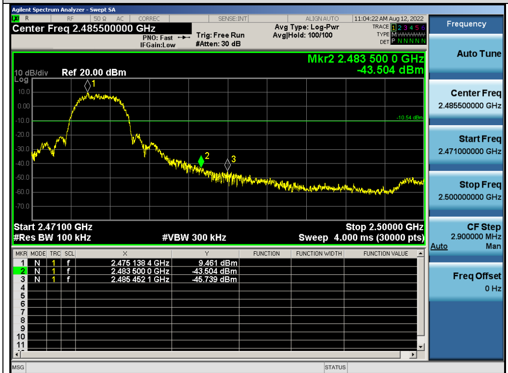
Test_Graph_GFSK_ANT1_2476_Higher Band Edge Emissions
