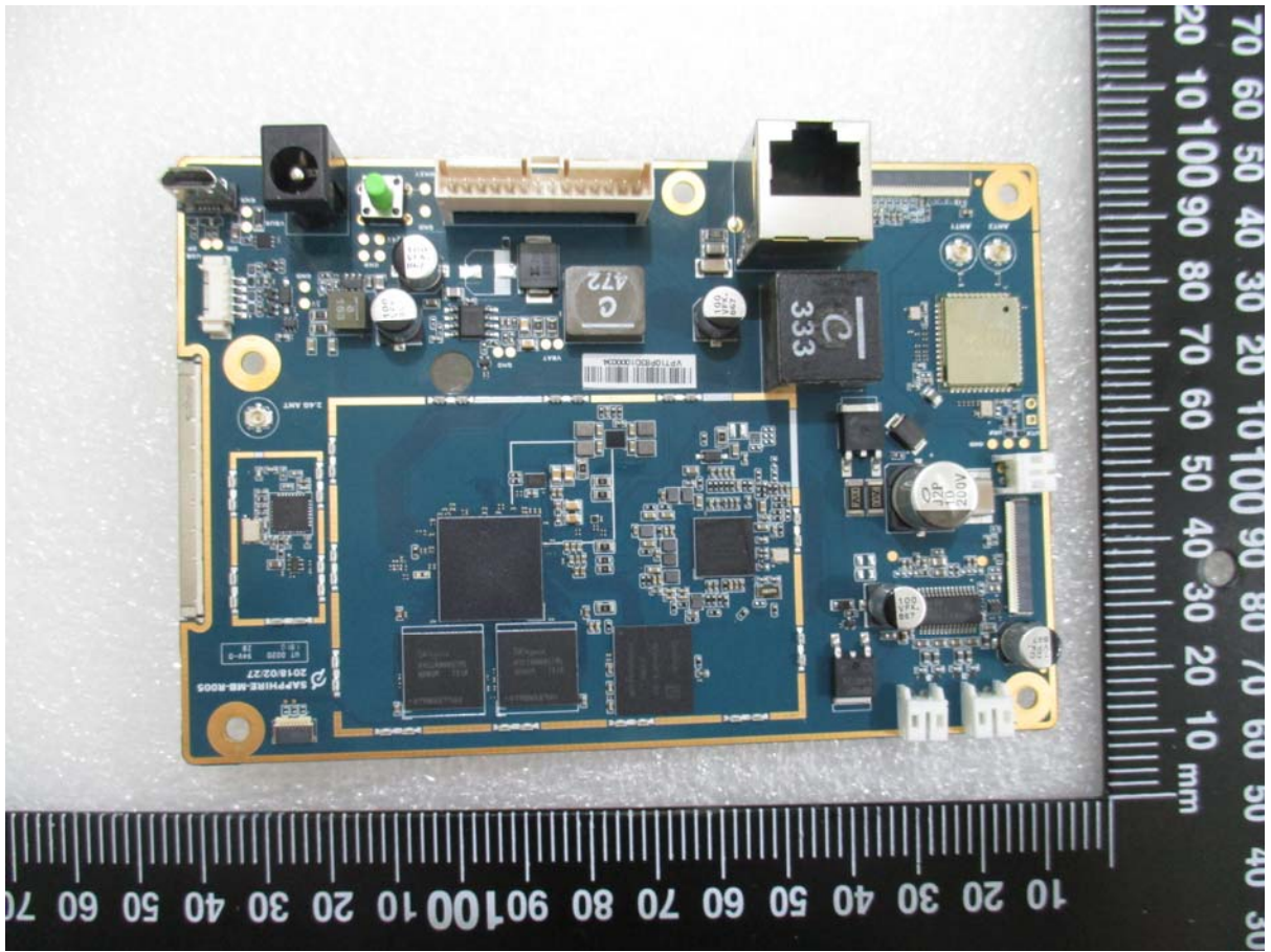
WiFi+BT+ANT+ module
