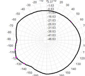
5500.0MHz Total(H-XY) Max= 0.26dBi
