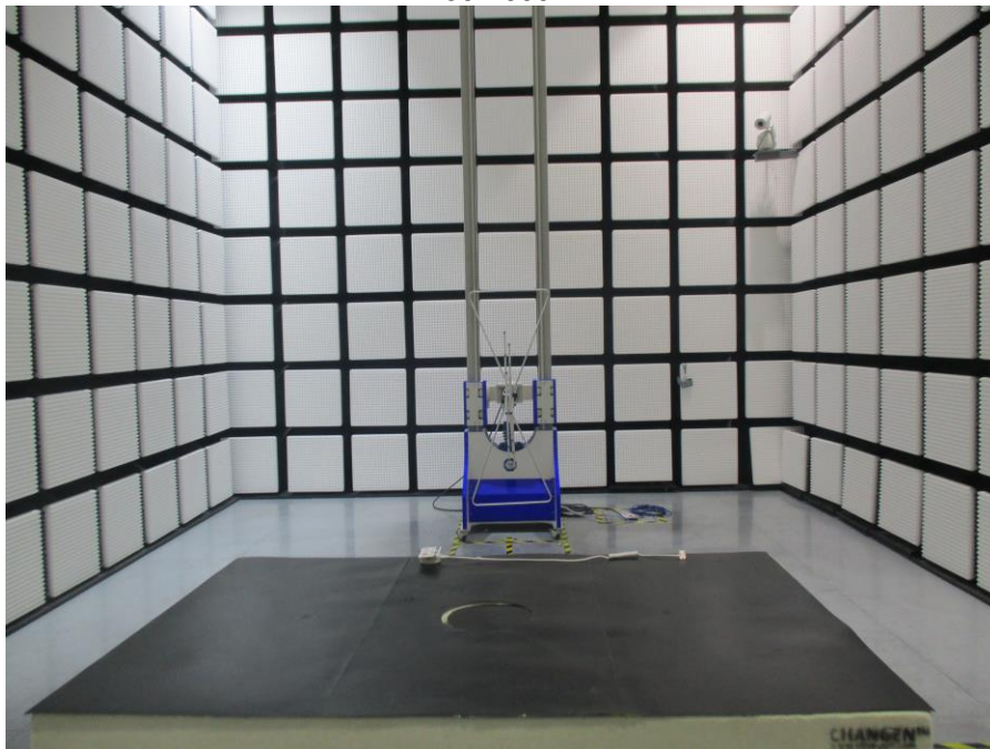
RE 30-1000MHz
