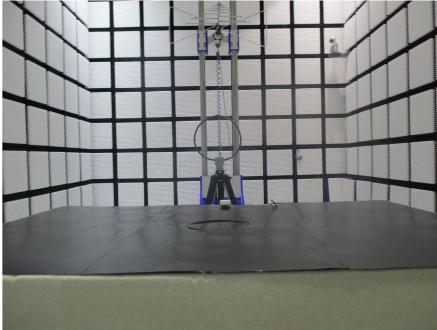
RE 30-1000MHz
