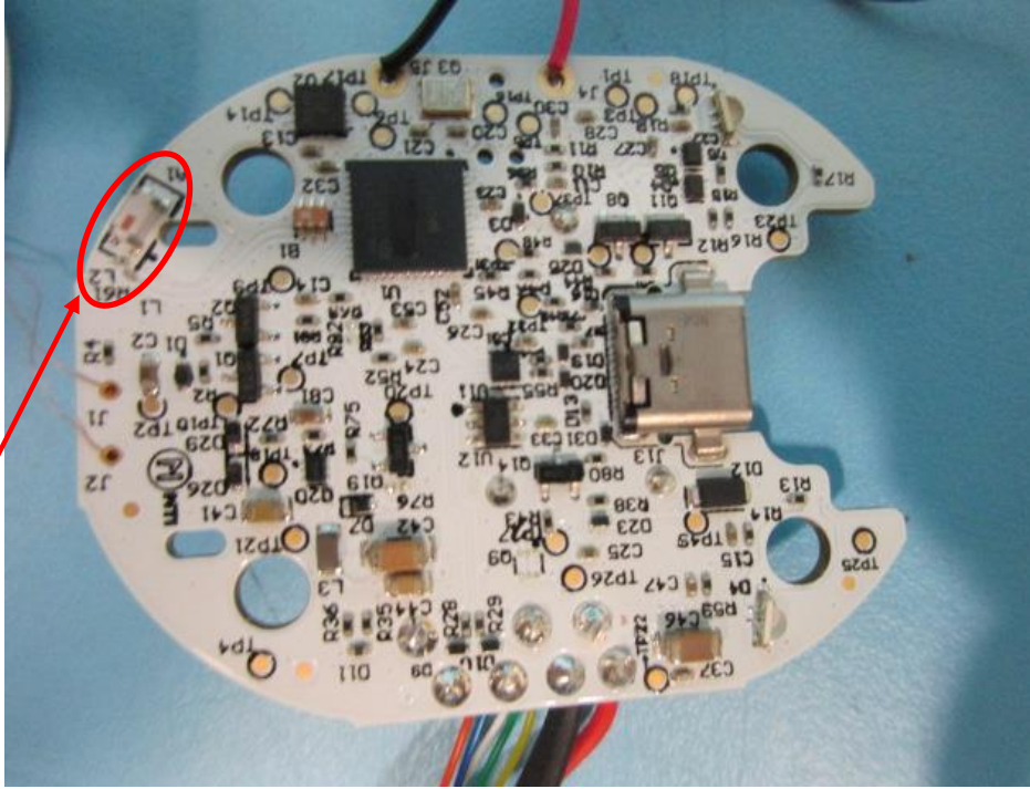
2.4GHz Antenna
