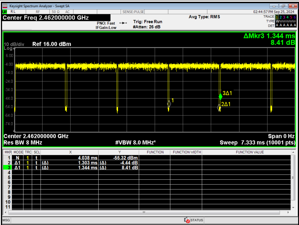
IEEE 802.11n_20MHz_Channel 11
