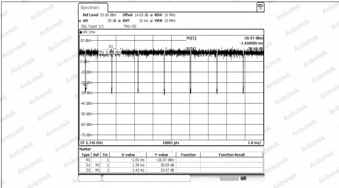
NTNV-11A-Ant1-5745
