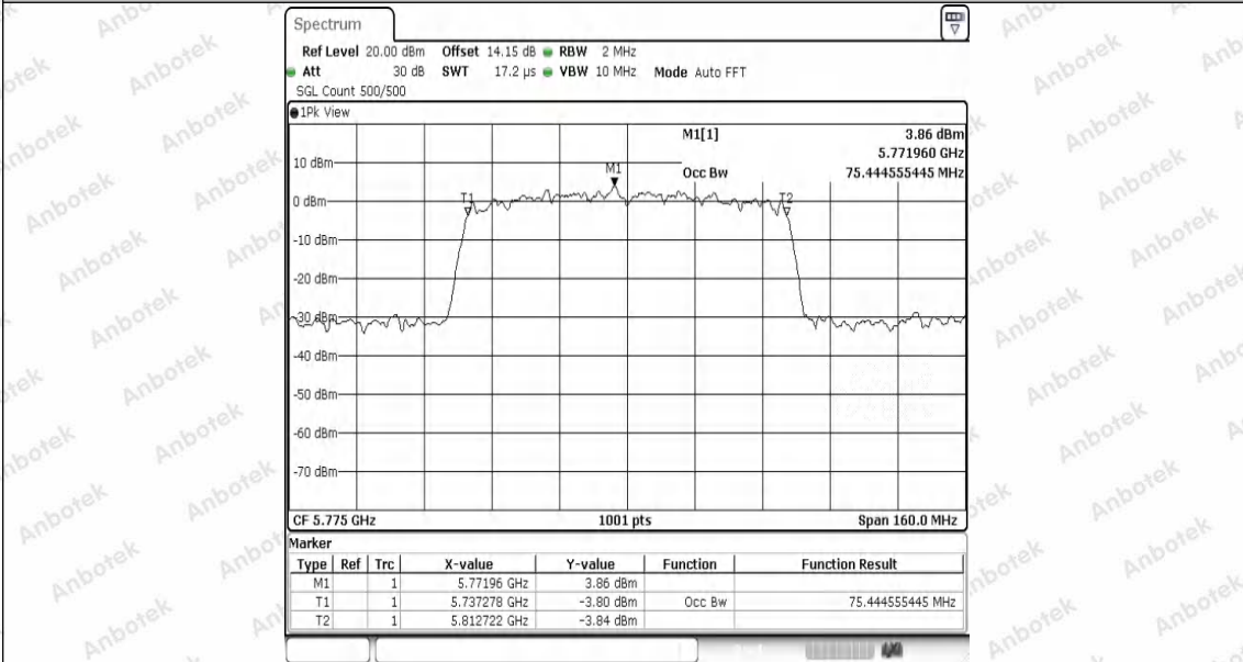
11AC80SISO-Ant1-5775
