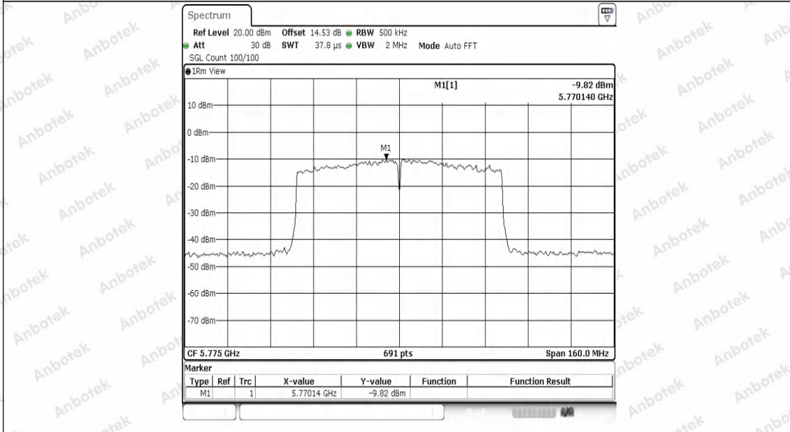
11AC80SISO-Ant1-5775-PASS
