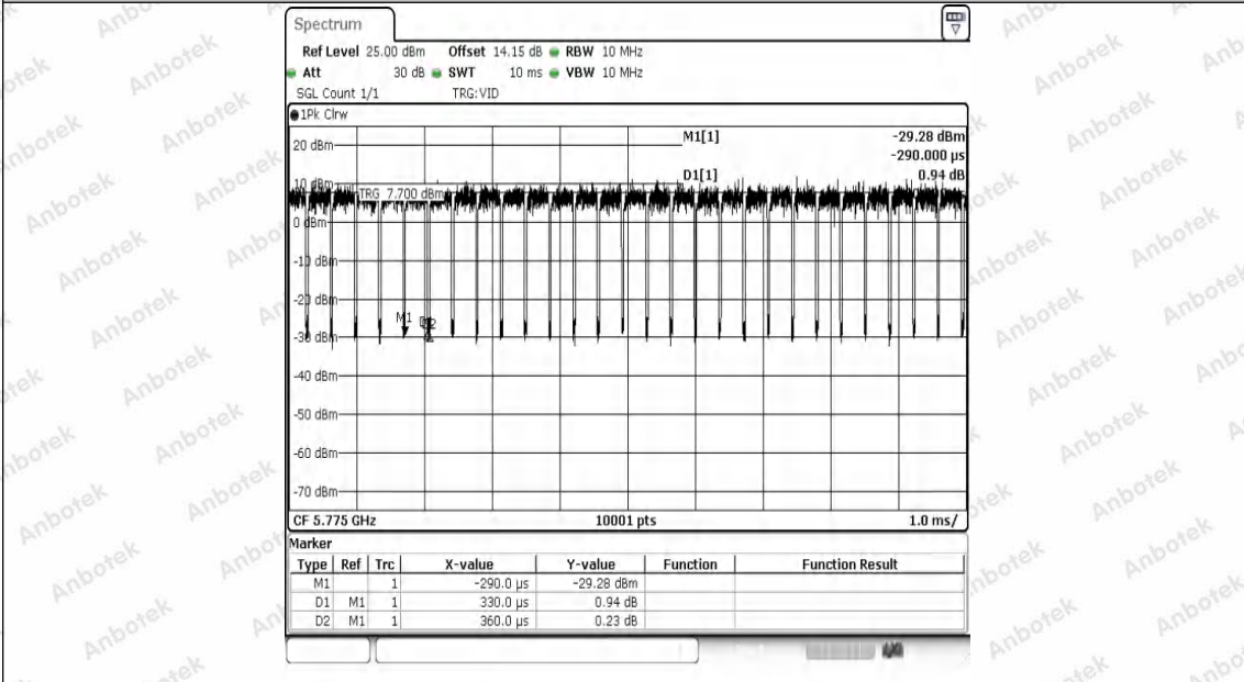
NTNV-11AC80SISO-Ant1-5775
