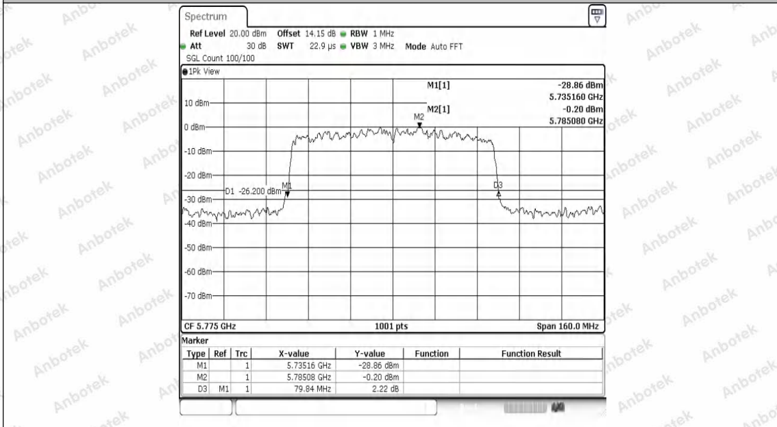
11AC80SISO-Ant1-5775
