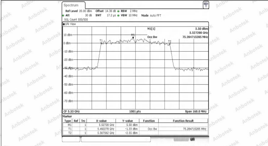
11AC80SISO-Ant1-5530
