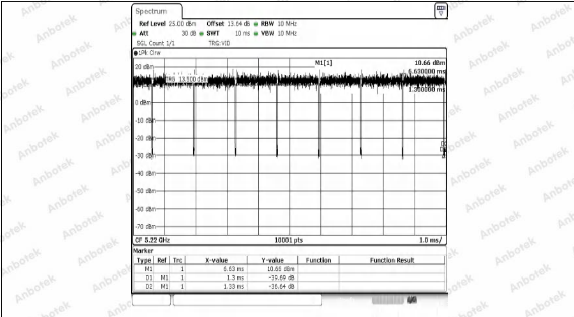
NTNV-11N20SISO-Ant1-5220
