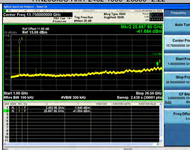
11N20SISO-Ant1-2462-1000~26500--2.22
