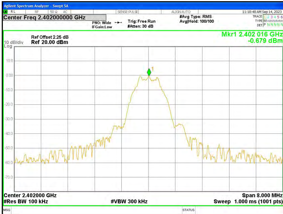
Band Edge NVNT BLE 1M 2402MHz Ant3 Ref
