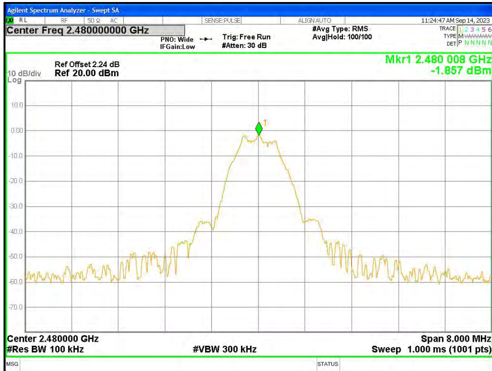
Band Edge NVNT BLE 1M 2480MHz Ant3 Ref
