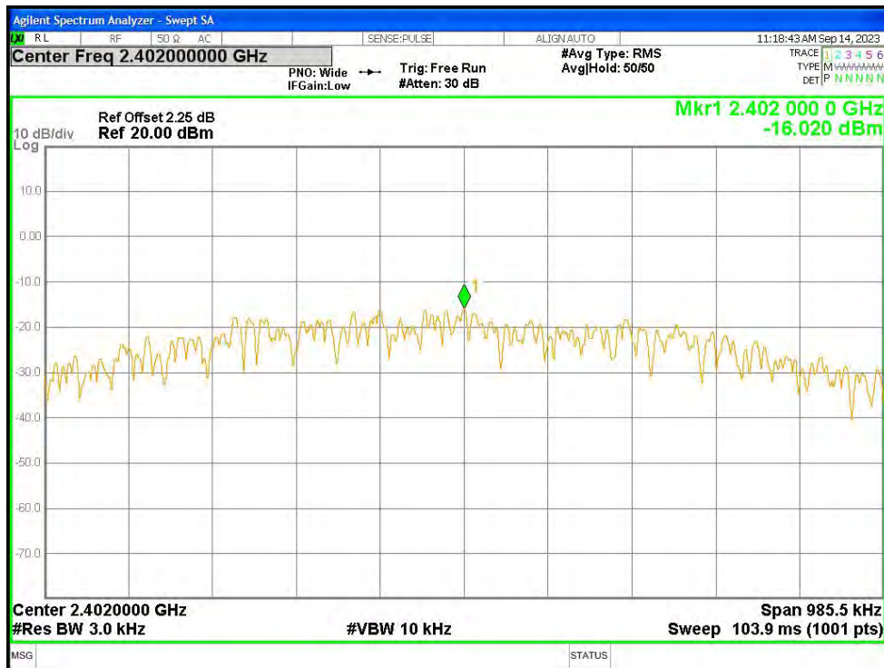
PSD NVNT BLE 1M 2402MHz Ant3
