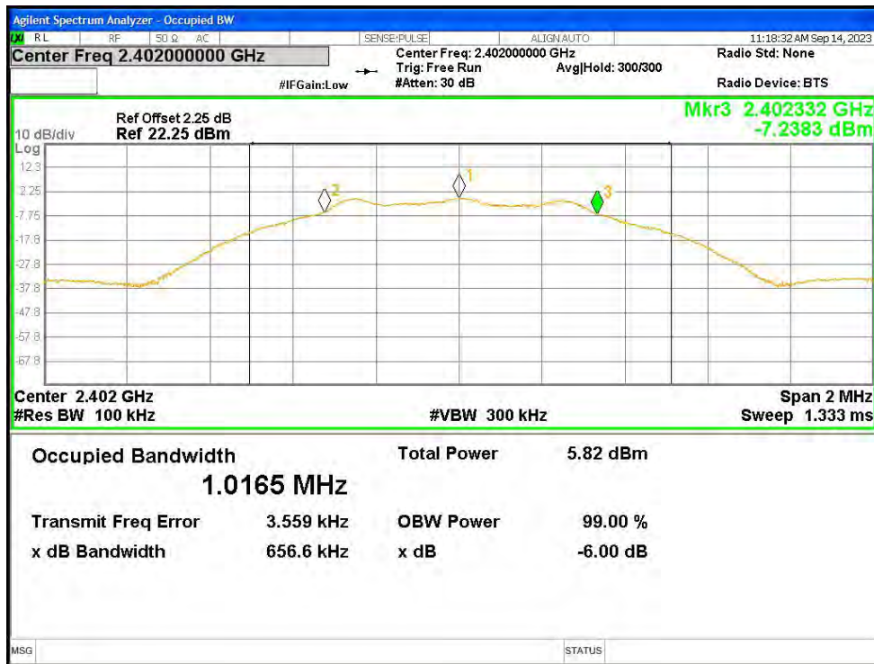
-6dB Bandwidth NVNT BLE 1M 2402MHz Ant3
