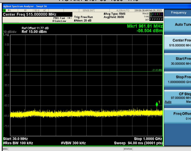
11G-Ant1-2437-30~1000--1.43
