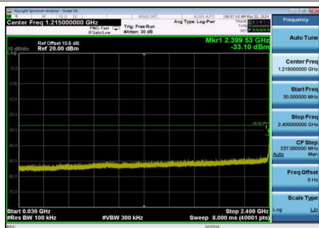
,Plot 3,30MHz~2400MHz-802.11g,2462MHz
