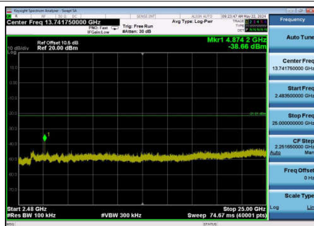
,Plot 4,2483.5MHz~25000MHz-802.11b
