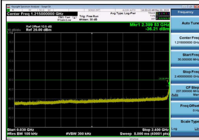
,Plot 3,30MHz~2400MHz-802.11n(40MHz) ,2452MHz,Ant0
