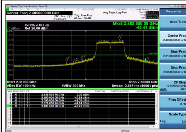
,Plot 2,Band Edge-802.11n(40MHz) ) ,2437MHz,Ant0
