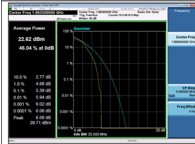
Band25-20MHz-16QAM-26365-1RB#0-PASS
