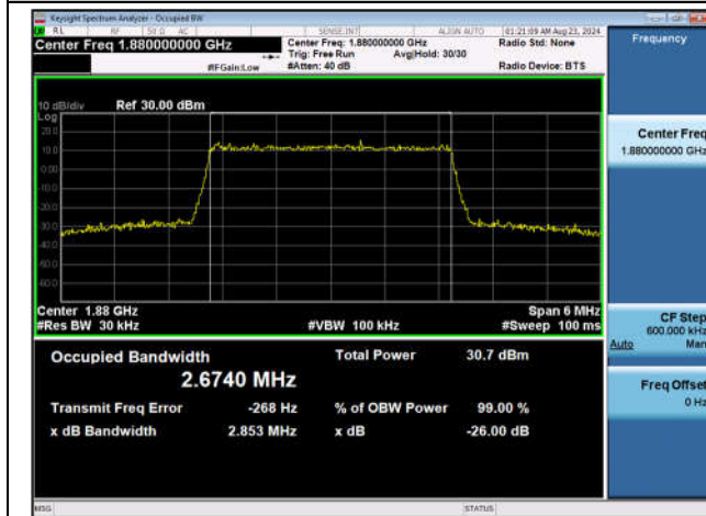
Band2-3MHz-QPSK-18900-15RB#0-PASS
