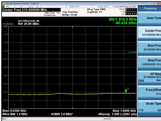
Band4-1312-30~1000MHz-PASS
