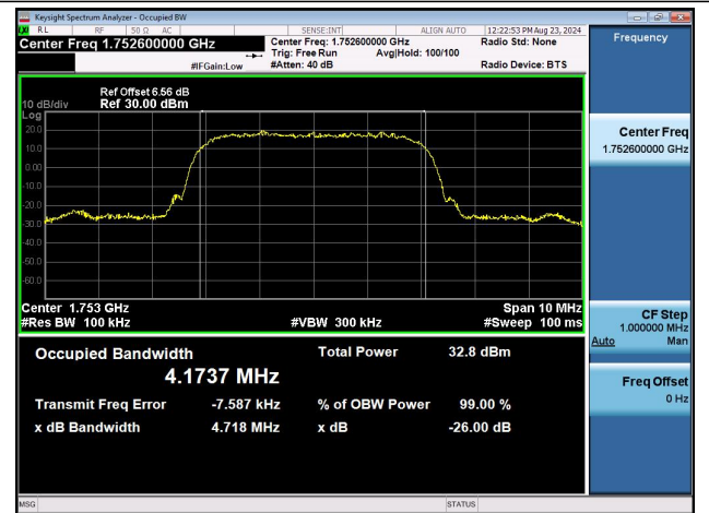
Band4-1513-PASS
