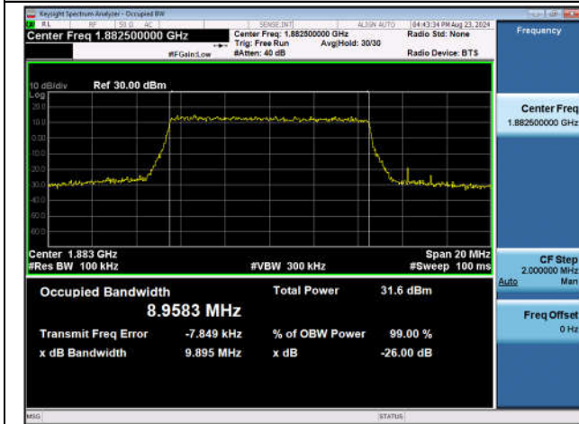
Band25-10MHz-QPSK-26365-50RB#0-PASS
