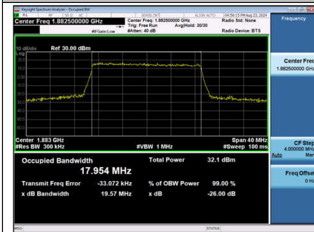
Band25-20MHz-QPSK-26365-100RB#0-PASS
