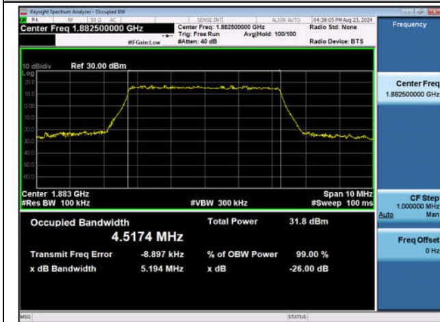
Band25-5MHz-QPSK-26365-25RB#0-PASS
