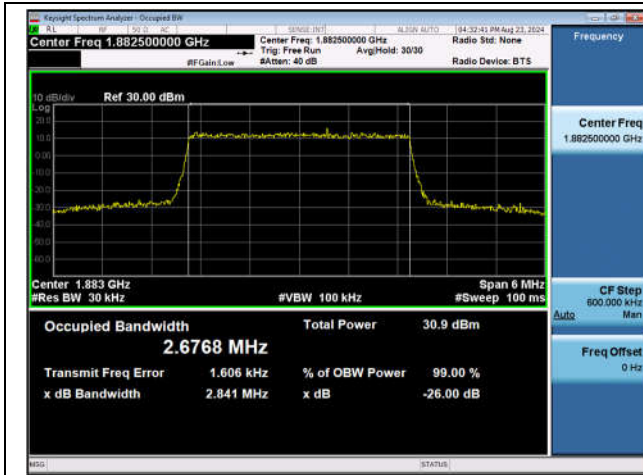
Band25-3MHz-QPSK-26365-15RB#0-PASS
