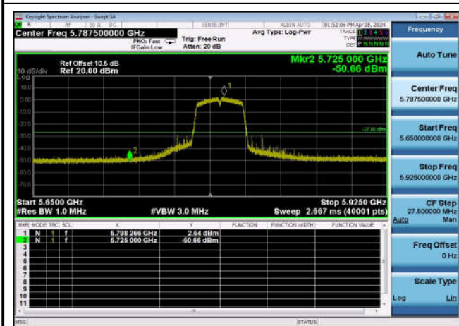
U-NII-3 ,Plot 1,Band Edge-802.11ac(40 MHz),5795MHz,Ant1
