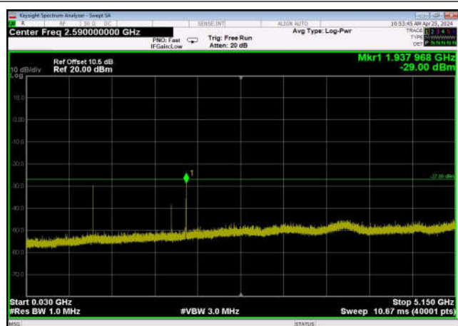
U-NII-1 ,Plot 2,30MHz~5150MHz-802.11a c(20MHz),5180MHz,Ant1
