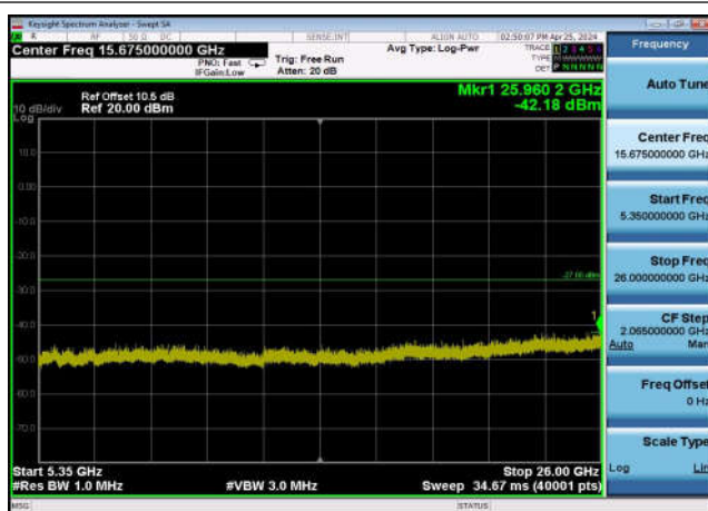
U-NII-1 ,Plot 3,5350MHz~26000MHz-802. 11ac(40MHz),5190MHz,Ant1
