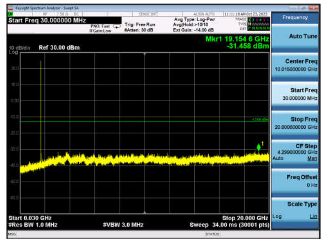
N66_40MHz_DFT-s-OFDM_BPSK_ Edge_1RB_Left_Low_CH
