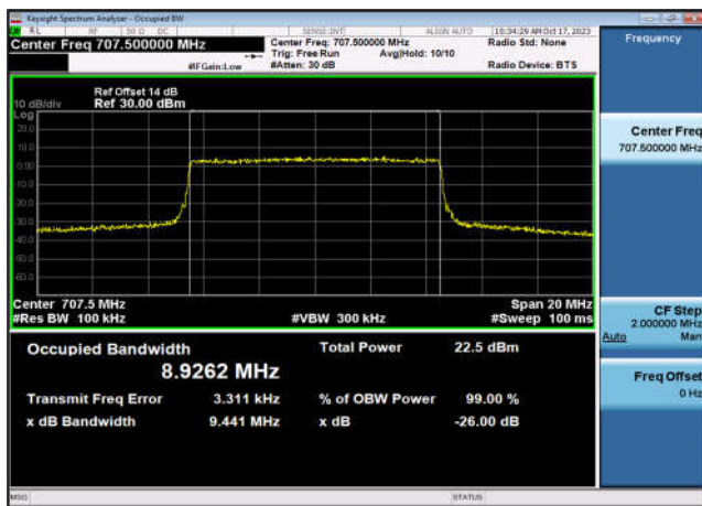
FDD12_MidRange_3_707.5_Q16
