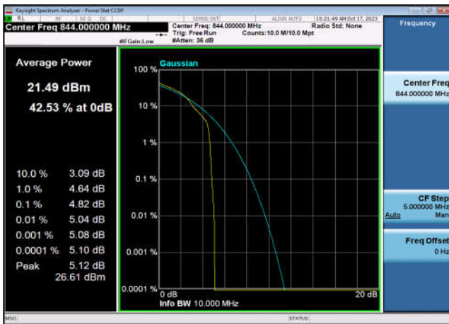
FDD26_Part 22_HighRange_10MHz_844_OneRB_high_Q16
