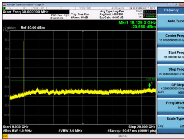
PCS 1900-810, 30MHz ~20GHz
