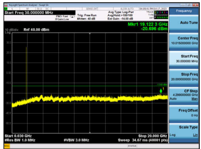
EGPRS 1900-810, 30MHz ~20GHz
