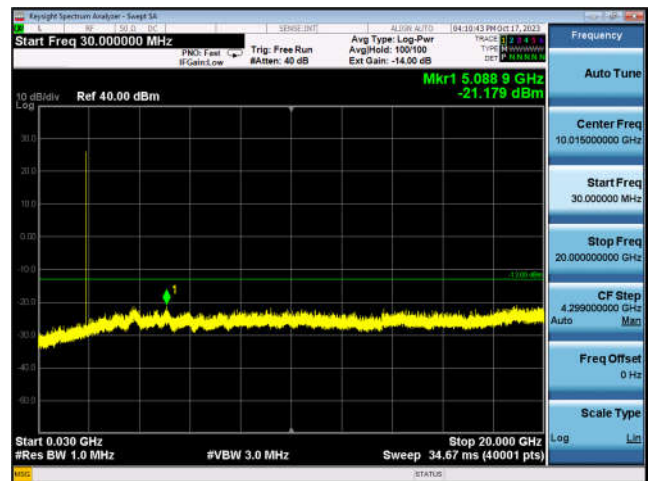
EGPRS 1900-810, 30MHz ~20GHz
