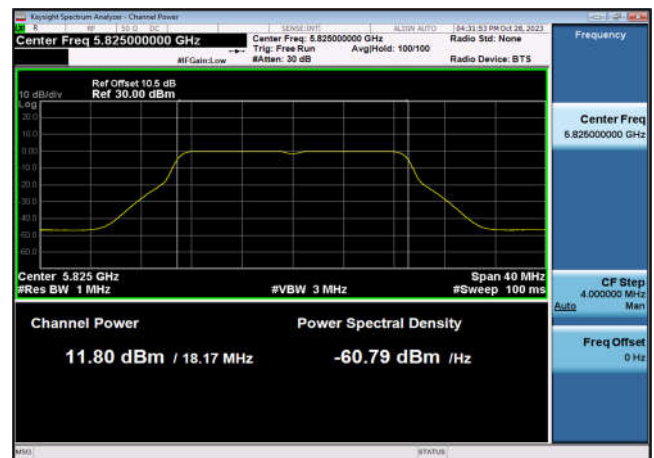
U-NII-3 Output Power-802.11n(20MHz) ,5825MHz,Ant6
