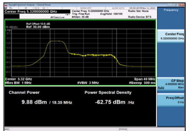
U-NII-2a Output Power-802.11ax(20MHz _RU52_1),5320MHz,Ant6
