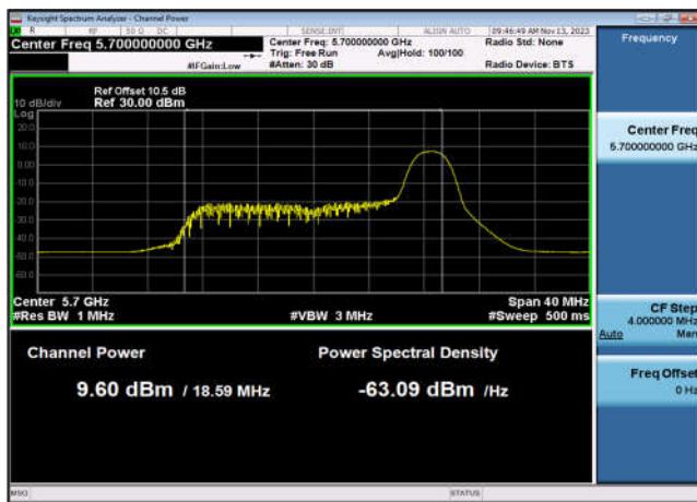
U-NII-2c Output Power-802.11ax(20MHz _RU26_9),5700MHz,Ant7
