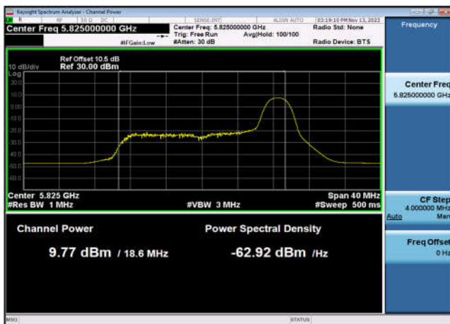
U-NII-3 Output Power-802.11ax(20MHz _RU26_9),5825MHz,Ant7
