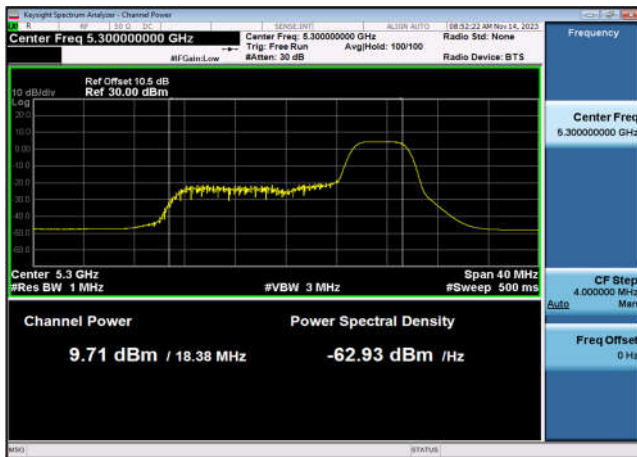
U-NII-2a Output Power-802.11ax(20MHz _RU52_4),5320MHz,Ant7
