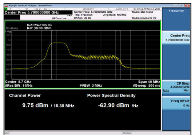
U-NII-2c Output Power-802.11ax(20MHz _RU52_1),5700MHz,Ant6
