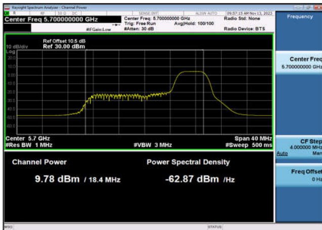
U-NII-2c Output Power-802.11ax(20MHz _RU52_4),5700MHz,Ant7
