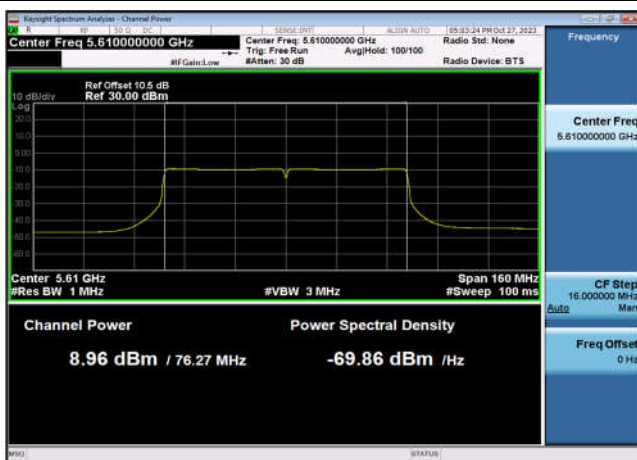
U-NII-2c Output Power-802.11ac(80MHz) ,5610MHz,Ant7
