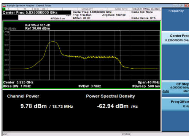
U-NII-3 Output Power-802.11ax(20MHz _RU26_1),5825MHz,Ant7
