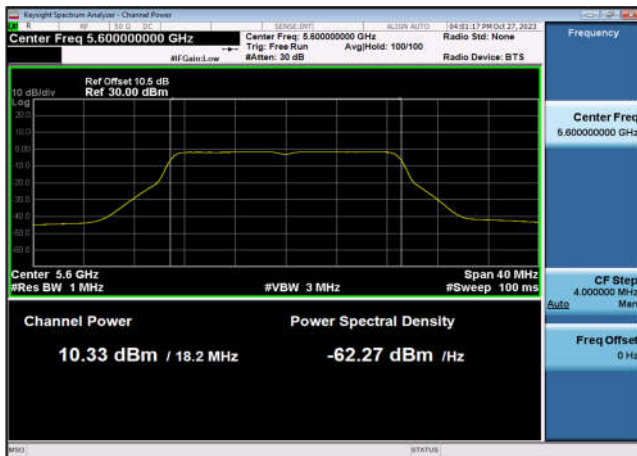
U-NII-2c Output Power-802.11ac(20MHz) ,5600MHz,Ant7
