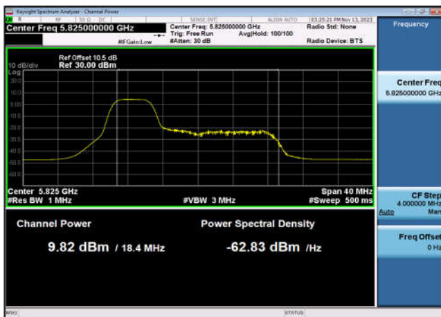
U-NII-3 Output Power-802.11ax(20MHz _RU52_1),5825MHz,Ant7
