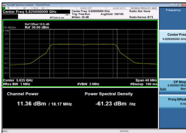
U-NII-3 Output Power-802.11n(20MHz) ,5825MHz,Ant7
