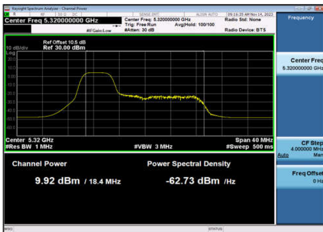
U-NII-2a Output Power-802.11ax(20MHz _RU52_1),5320MHz,Ant7
