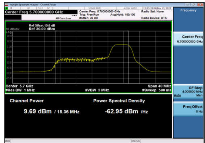
U-NII-2c Output Power-802.11ax(20MHz _RU52_4),5700MHz,Ant6
