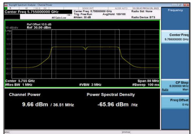
U-NII-3 Output Power-802.11ac(40MHz) ,5755MHz,Ant6
