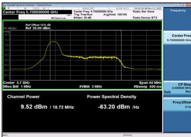
U-NII-2c Output Power-802.11ax(20MHz _RU26_1),5700MHz,Ant7
