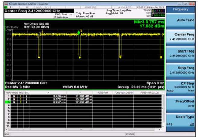
DutyCycle-802.11ax(HE20_RU26_1) ,2412MHz,Ant7
