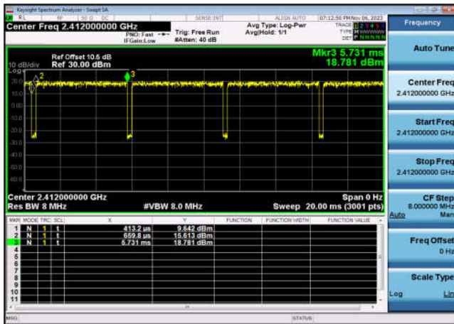
DutyCycle-802.11ax(HE20_RU52_1) ,2412MHz,Ant7
