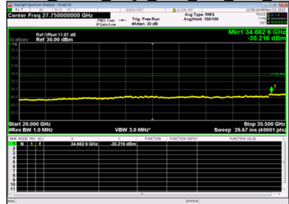
n77(40M)_DFT-s-OFDM QPSK Edge 1RB Left Low CH
