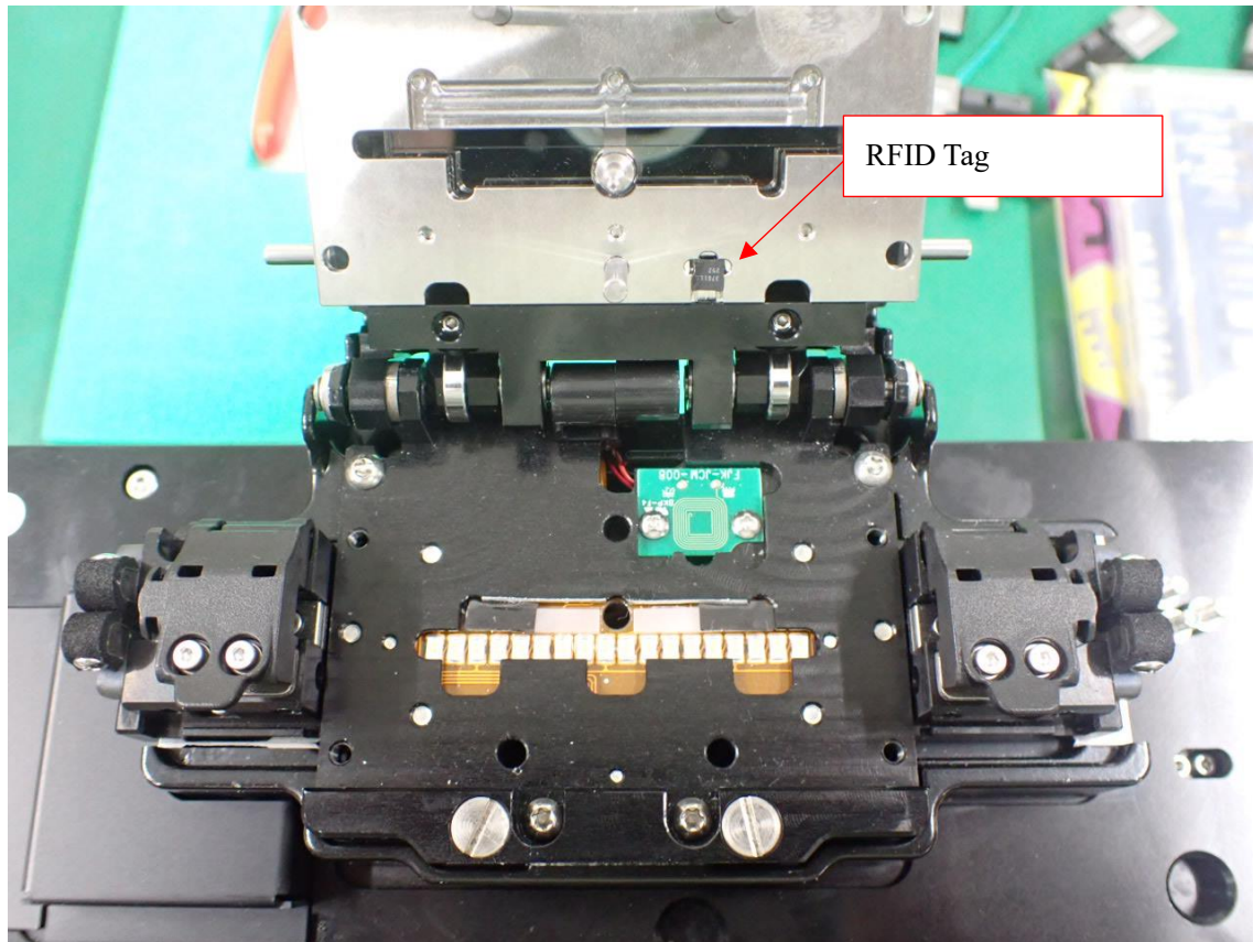
RFID Tag
