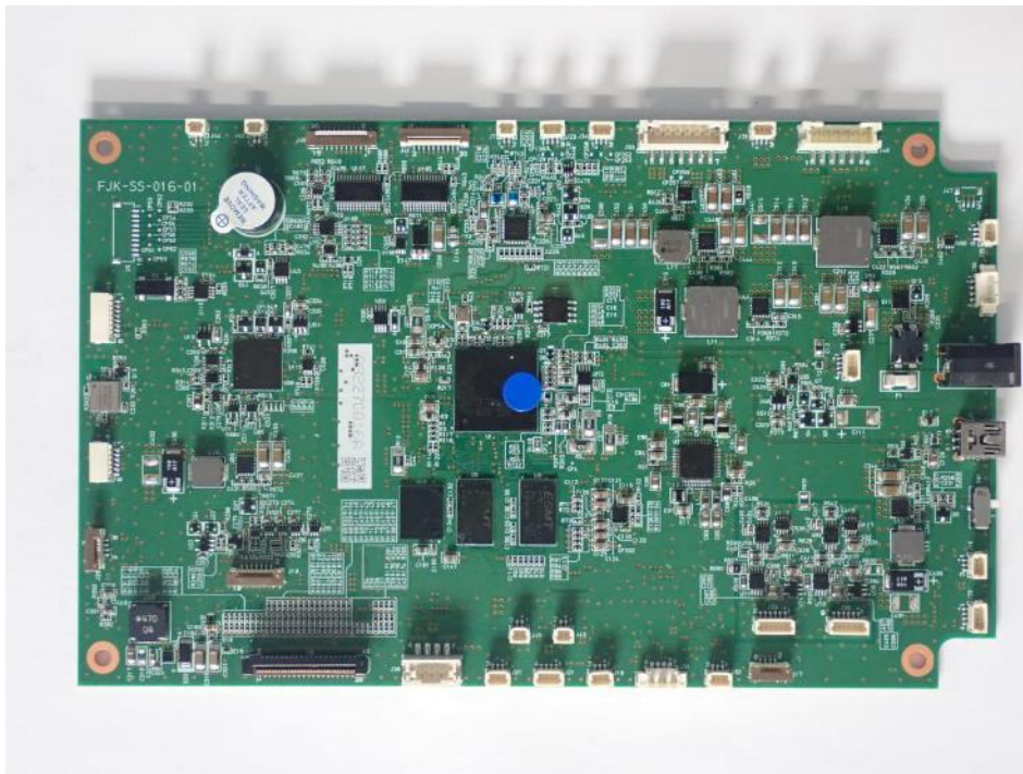
Mianboard (Front)
