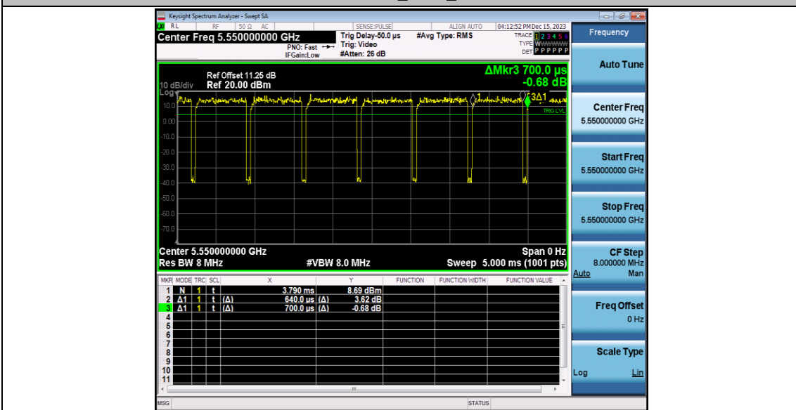
11N40SISO_Ant 0_5550
