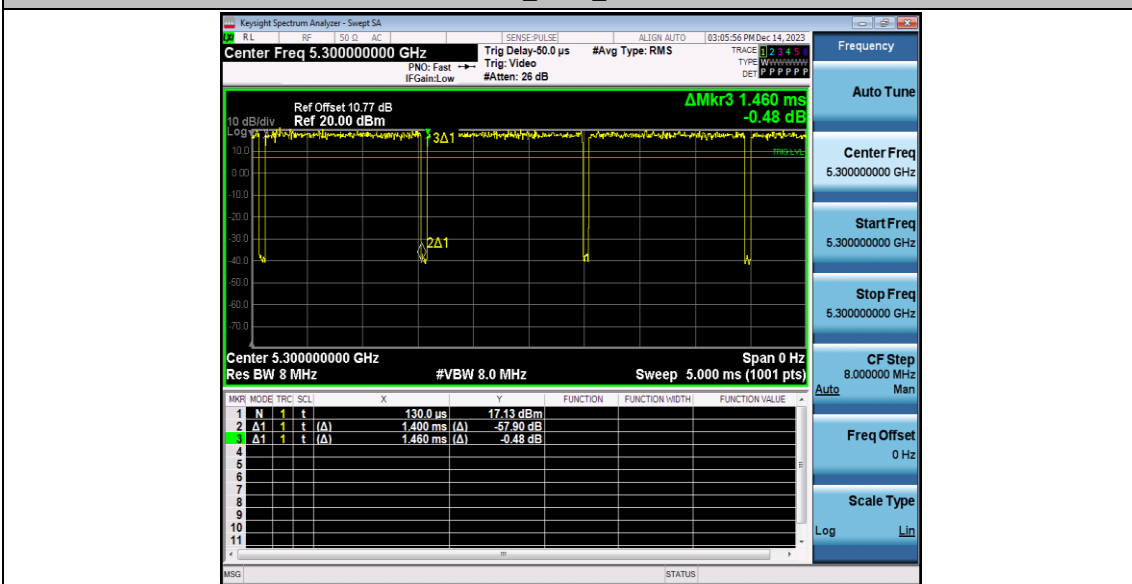
11A_Ant 0_5300
