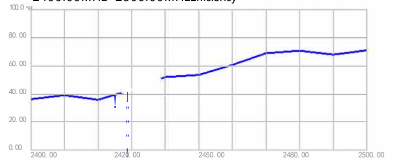
2400.00MHz- 2500.00MHzEfficiency
