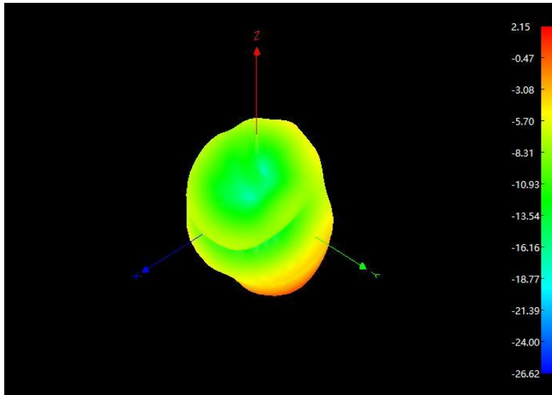
2500MHz 3D
