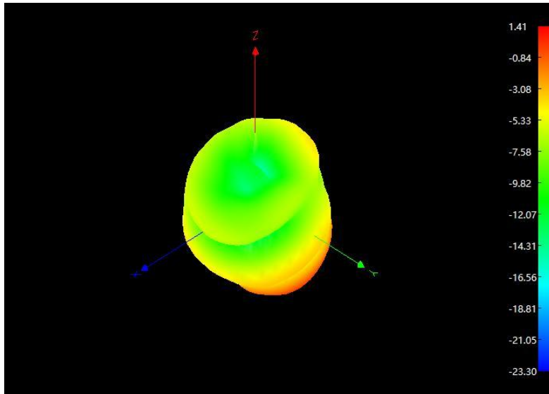
2450MHz 3D
