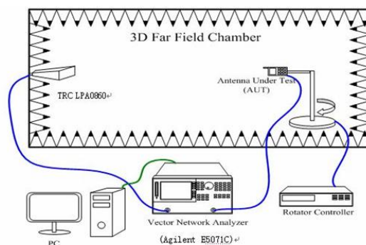
图 1. 微波暗室内部仪器设置 r.4
