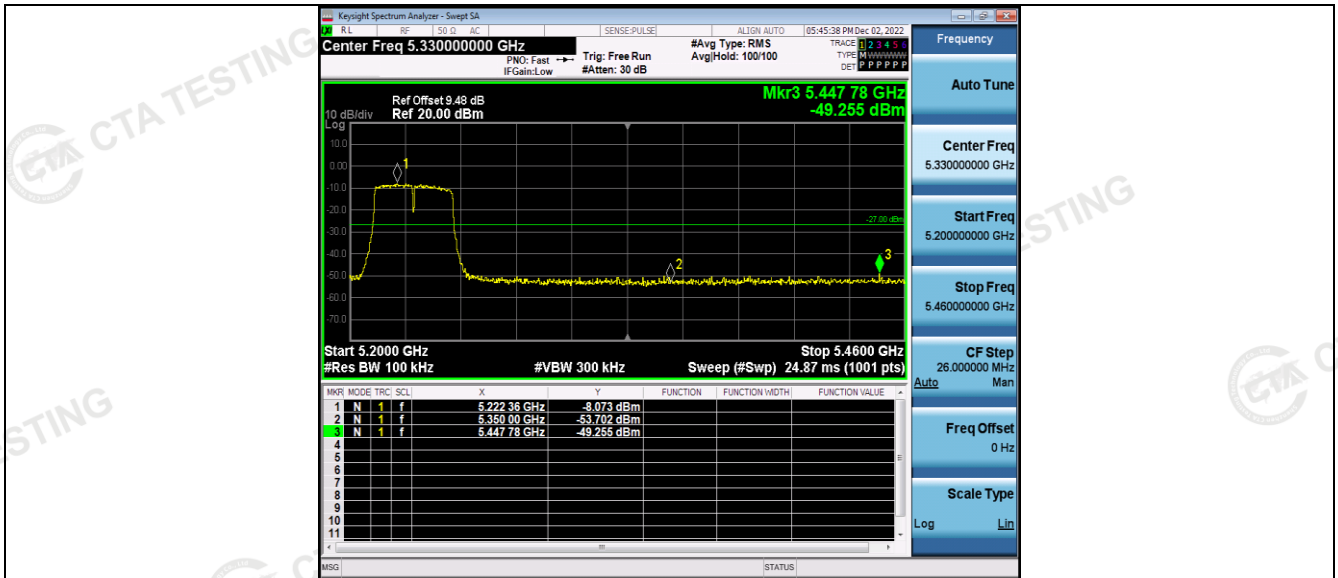
11AC80SISO_Ant1_Low_5210
