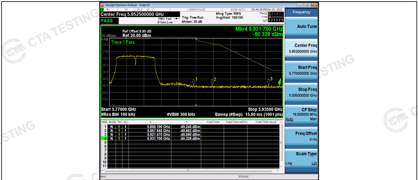
11AC80SISO_Ant1_Low_5775
