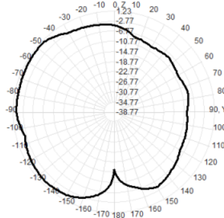
2450.0MHz Total(E2-YZ), Max= 0.36dBi
