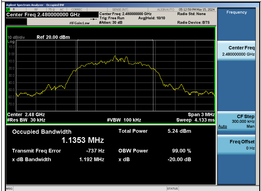
Test_Graph_EDR_ANT1_2480_3Mbps_OBW
