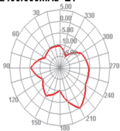
2400.000MHz E1
