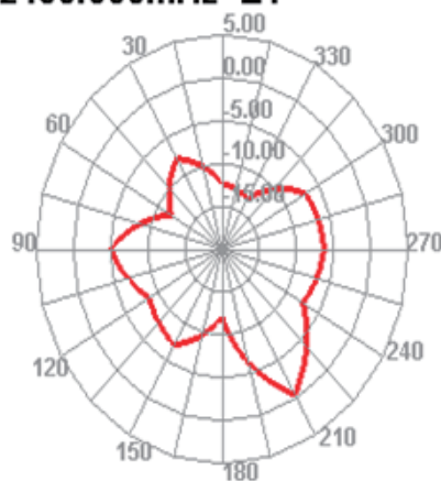
2450.000MHz E1
