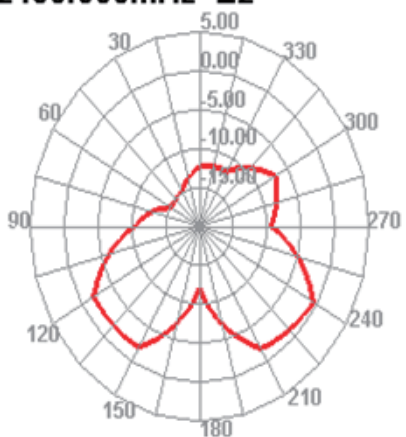
2450.000MHz E2
