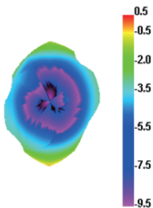
2450.000MHz
