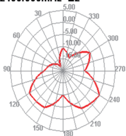
2400.000MHz E2
