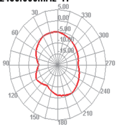
2450.000MHz H
